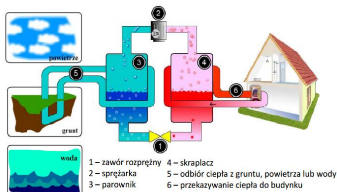
Rysunek 17 Zasada działania pompy ciepła 170
